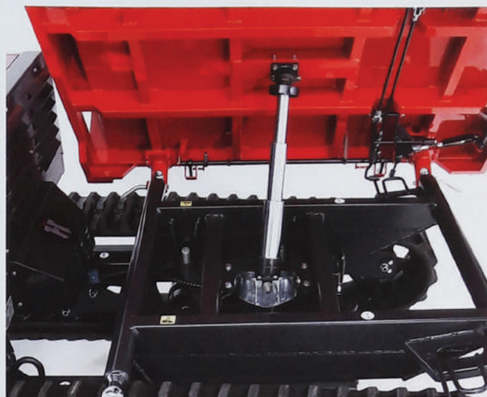
Oben: Der TX2500 ist ein kompaktes Raupenfahrzeug von Hinowa. Der Mechanismus zum Abkippen auf drei Seiten gelingt über einen Teleskopzylinder mit Gelenk (rechts).
